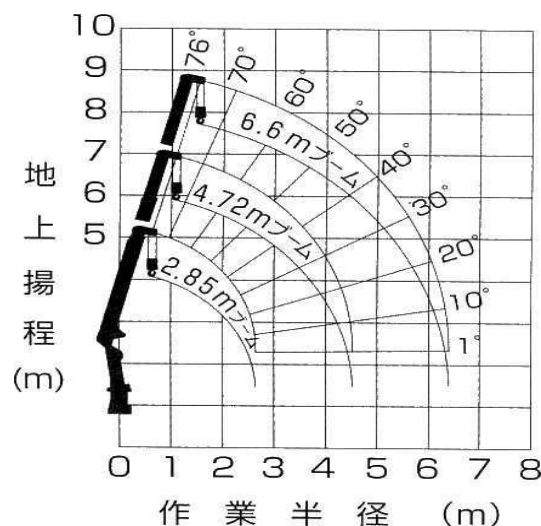
作業半径・揚程図
