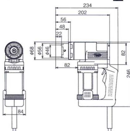
M20ソケット装着時寸法図
