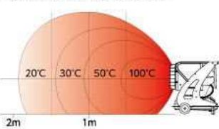
●温度分布図(上昇温度0℃基準)
