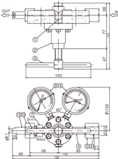
[外観寸法図]
