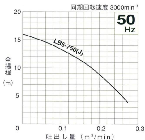
性能曲線
