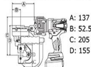
■壁からの穴あけ寸法図【単位：mm】
