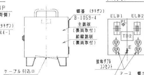
負荷側パネル
