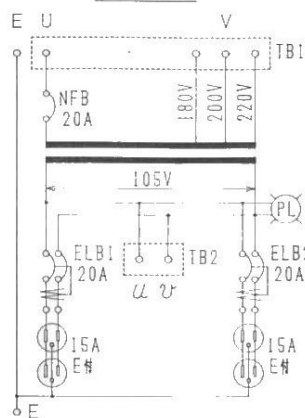
結線図
